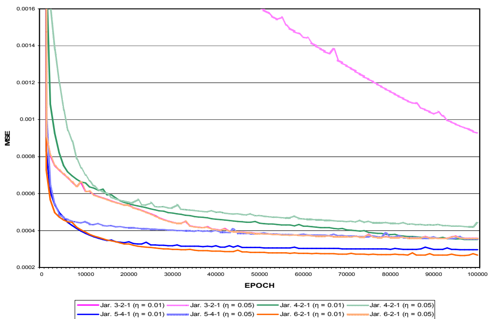
Gambar 3. Nilai MSE Hasil Pelatihan dengan Pengubahan Nilai Learning Rate ( \eta )
